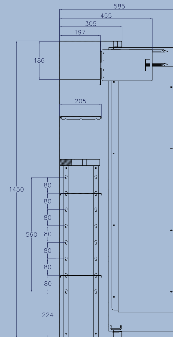
SECTION A-A
